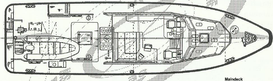
Maindeck
